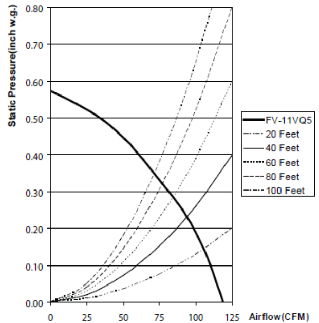
Fan Curve FV-11VQ5
