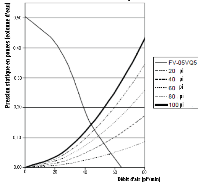
Courbe de rendement FV-05VQ5
