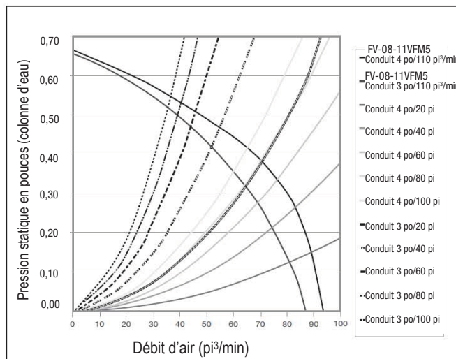
Courbe de rendement FV-08-11VFM5 - 110 pi³/min
