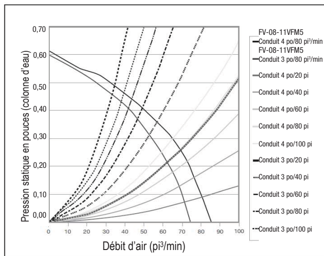
Courbe de rendement FV-08-11VFM5 - 80 pi³/min
