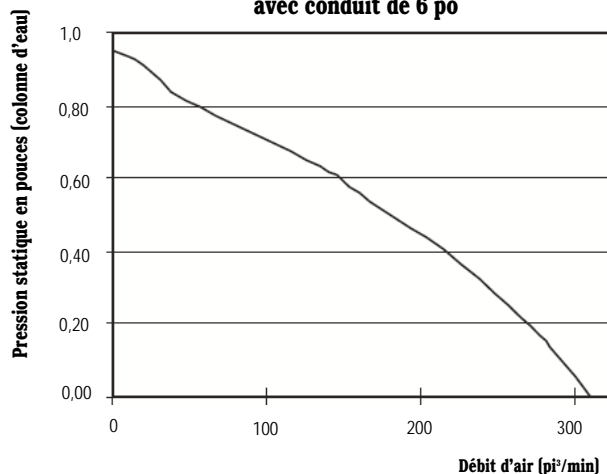
Courbe de rendement FV-30VQ3 avec conduit de 6 po
