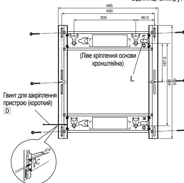
Вертикальний монтаж
